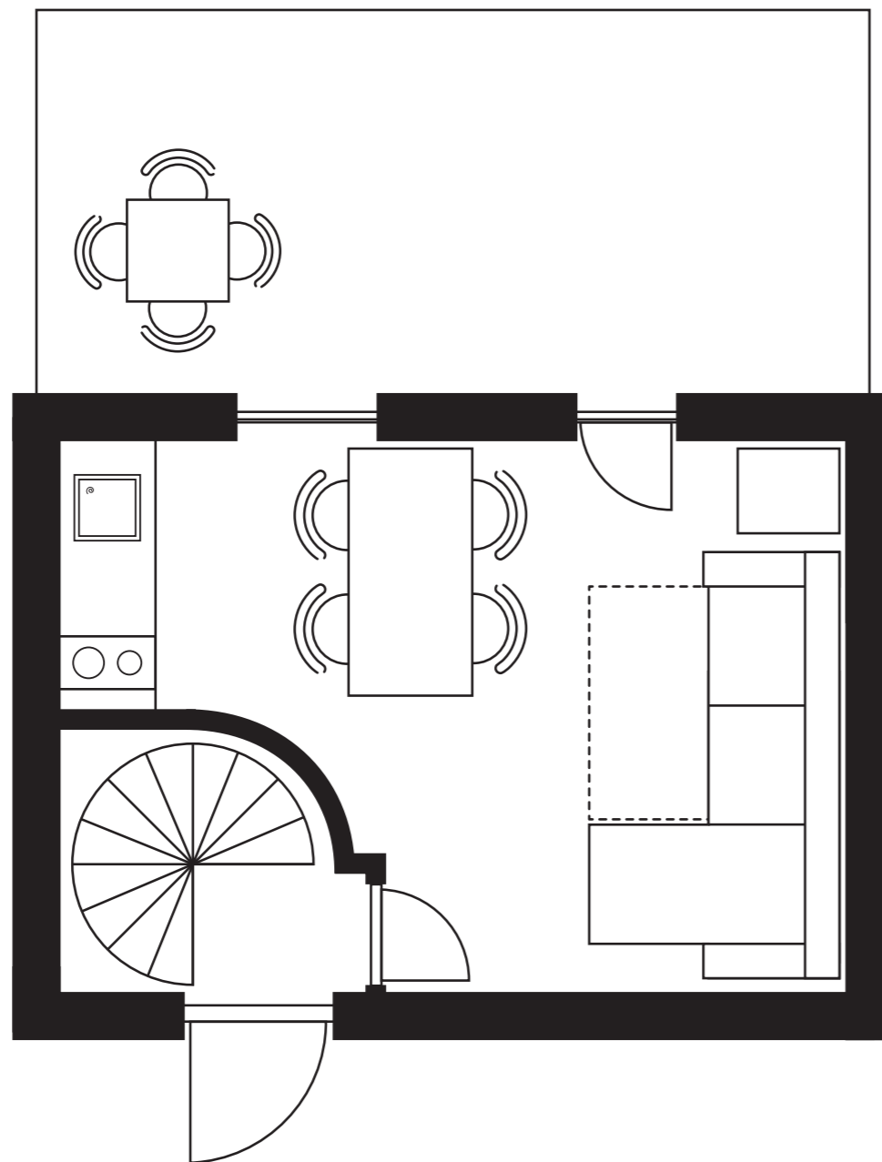
PRITLIČJE
